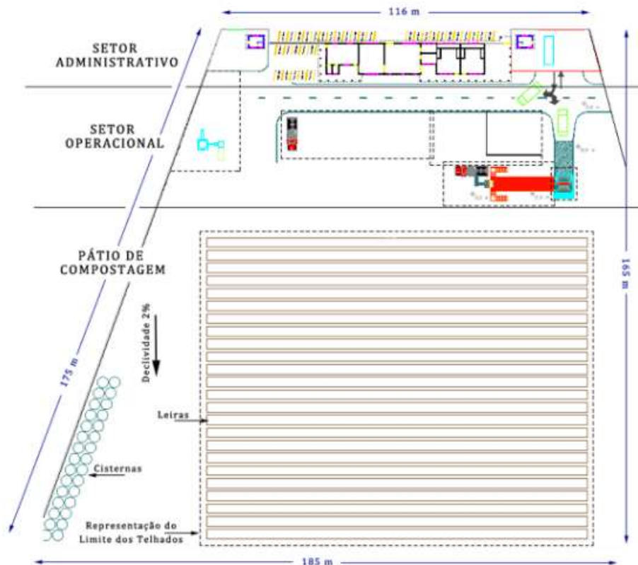
Figura 34 Plano técnico de una planta de compostaje de RSO (Análise econômica para implantação de uma usina de compostagem de resíduo orgânico urbano, 2017). 15
